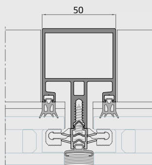
Sección Horizontal Fijos Sistema Mixto
