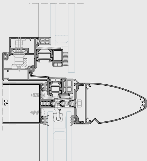
Sección Vertical Fijo con Proyectante
