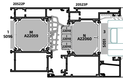
Accesorios sistema HQ - BALCONERA
