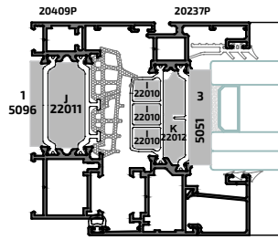
Accesorios sistema HQ - VENTANA
