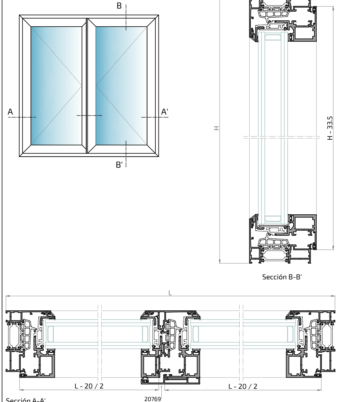
Sección A-A'
